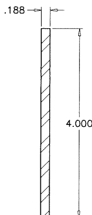
STIFFENER
