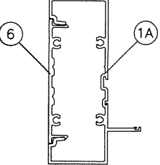
JAMB 'J1A'
