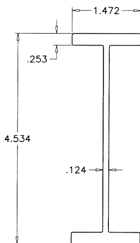
STIFFENER
